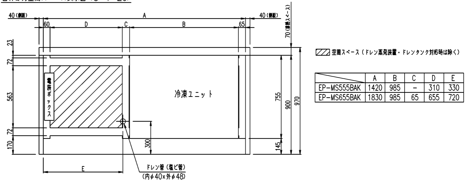
台枠部分空間スペース表示図 (S=1/20)
